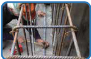
ΚΟΡΔΟΝΙ ΣΤΕΓΑΝΟΠΟΙΗΣΗΣ ΑΠΟ ΜΠΕΤΟΝΙΤΗ
