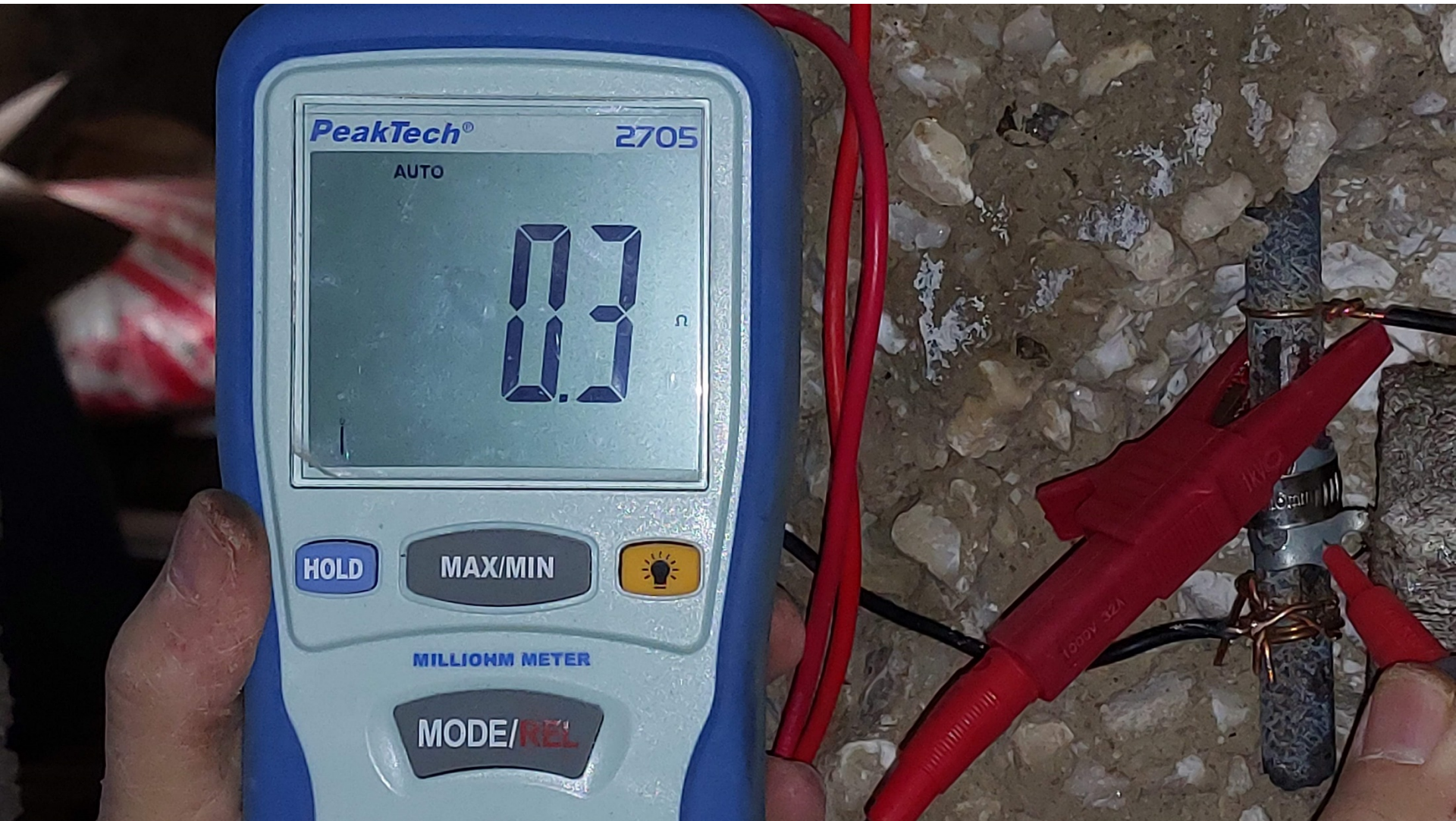
7. Μέτρηση σύνδεσης Ανοδίου και σπλισμού
